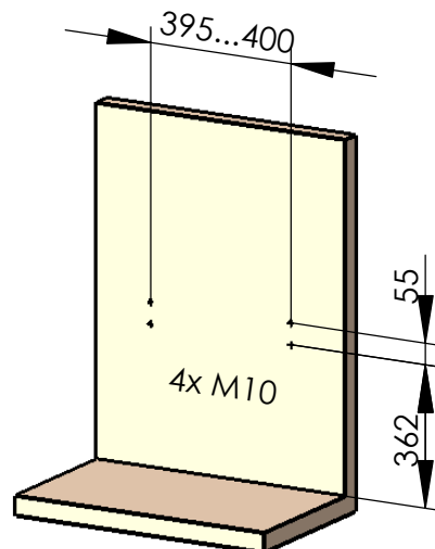
empfohlenes Lochbild
